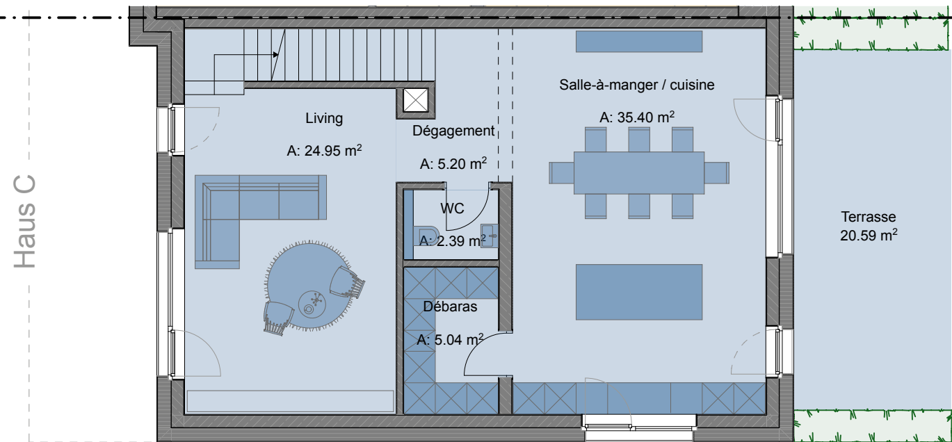
Rez-de-jardin
