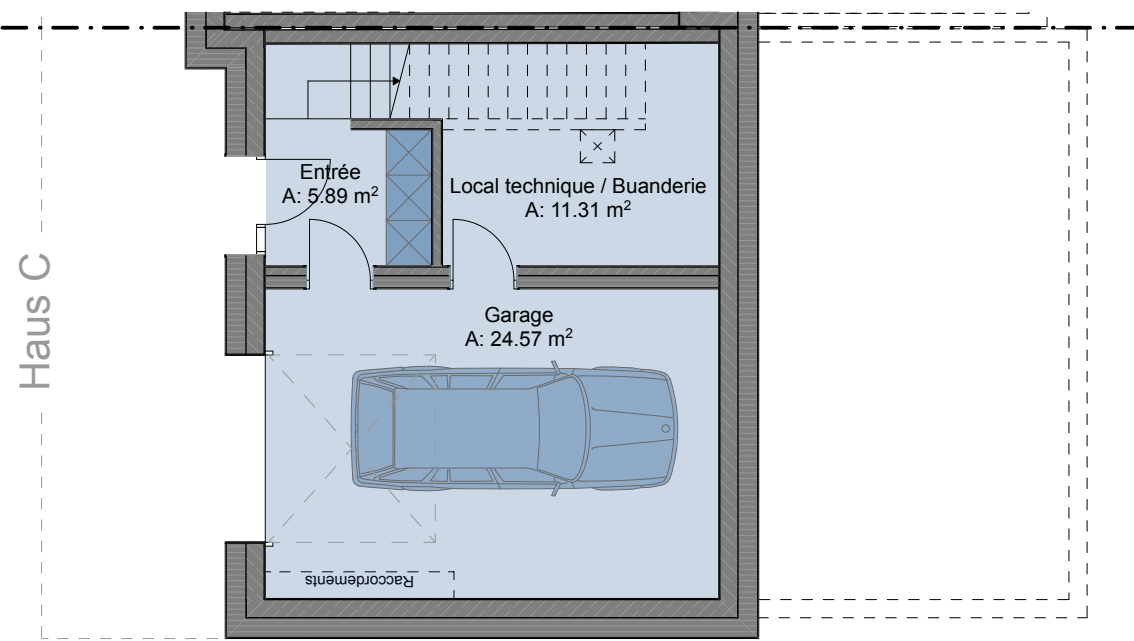
Rez-de-chaussée
