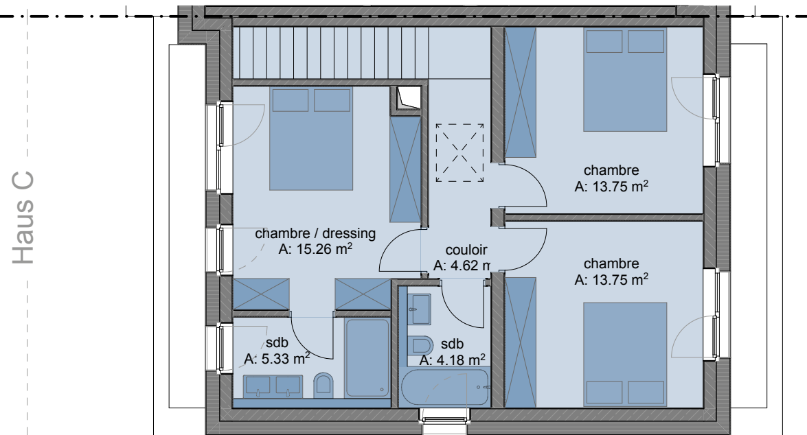
Etage +1
